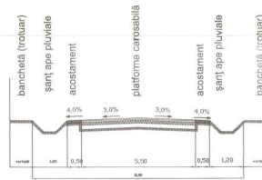
Secțiune caracteristică străzi reabilitate, 4,00 m
